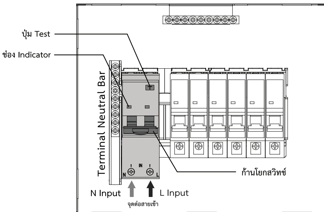
ภาพตัวอย่างการติดตั้งในตู้ Consumer Unit
